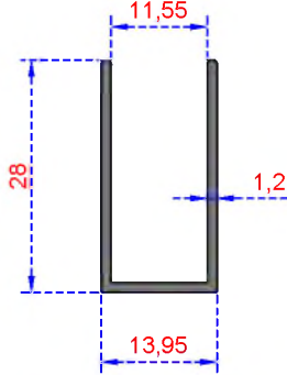
Sistem Kodu 1392 Ağırlık (kg/mt) 0,219
