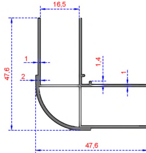
Sistem Kodu 2951 Ağırlık (kg/mt) 0,515
