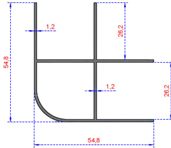
Sistem Kodu 2960 Ağırlık (kg/mt) 0,677
