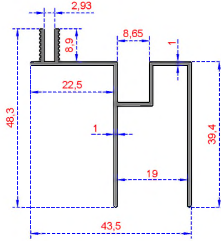
Sistem Kodu 2953 Ağırlık (kg/mt) 0,407
