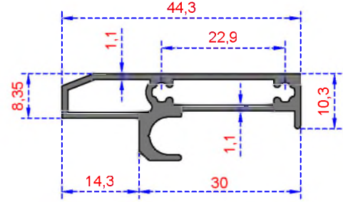
Sistem Kodu 2904 Ağırlık (kg/mt) 0,444
