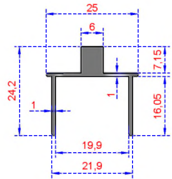
Sistem Kodu 2950 Ağırlık (kg/mt) 0,270
