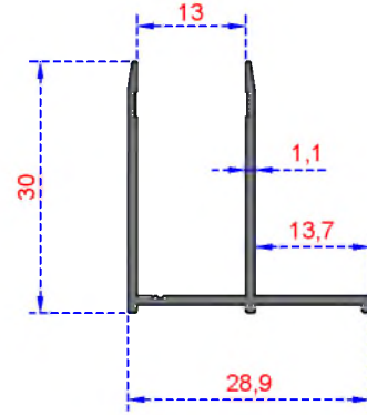
Sistem Kodu 2909 Ağırlık (kg/mt) 0,252
