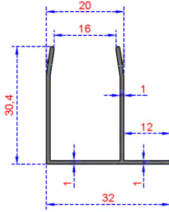
Sistem Kodu 2575 Ağırlık (kg/mt) 0,246
