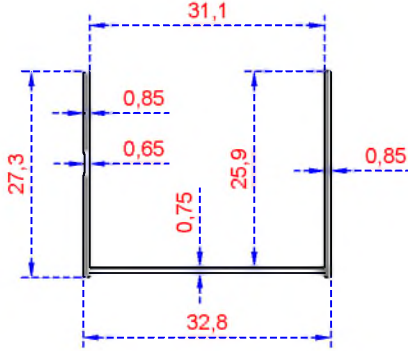
Sistem Kodu 2975 Ağırlık (kg/mt) 0,190
