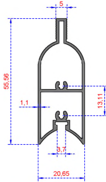
Sistem Kodu 2962 Ağırlık (kg/mt) 0,572
