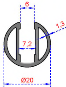
Sistem Kodu 1571 Ağırlık (kg/mt) 0,299
