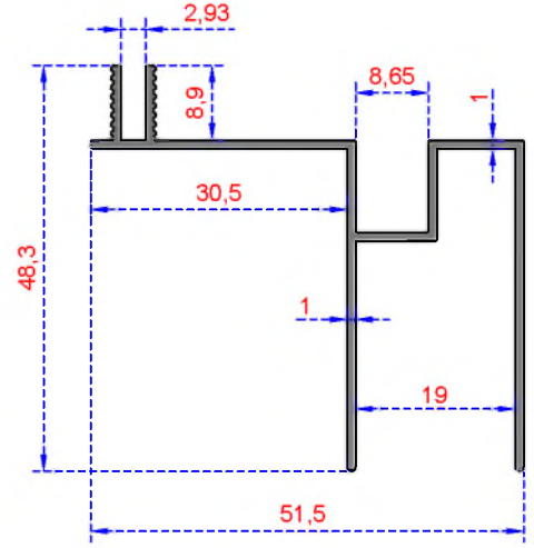
Sistem Kodu 2955 Ağırlık (kg/mt) 0,428
