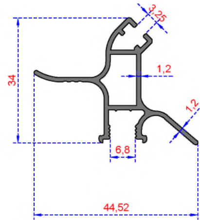
Sistem Kodu 1945 Ağırlık (kg/mt) 0,419
