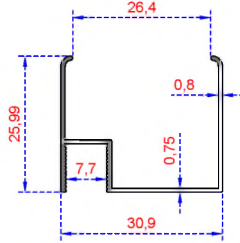
Sistem Kodu 2976 Ağırlık (kg/mt) 0,205
