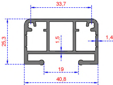
Sistem Kodu 2980 Ağırlık (kg/mt) 0,800
