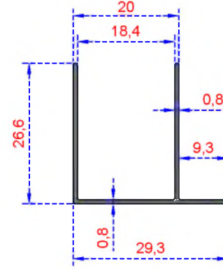
Sistem Kodu 2940 Ağırlık (kg/mt) 0,175
