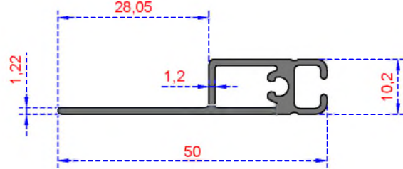
Sistem Kodu 1720 Ağırlık (kg/mt) 0,334
