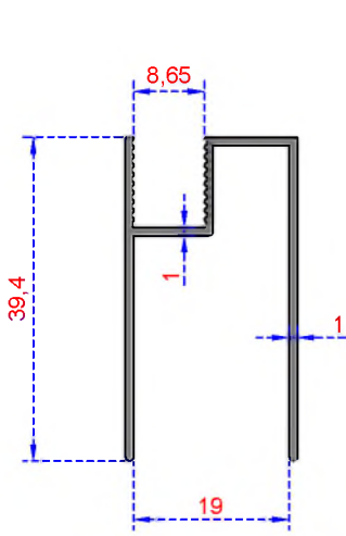
Sistem Kodu 2952 Ağırlık (kg/mt) 0,286
