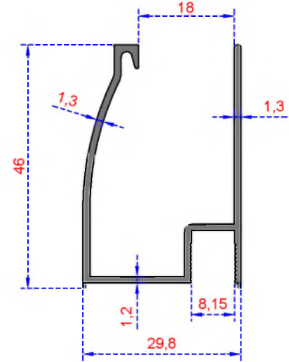
Sistem Kodu 2906 Ağırlık (kg/mt) 0,458
