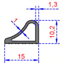
Sistem Kodu 2958 Ağırlık (kg/mt) 0,117
