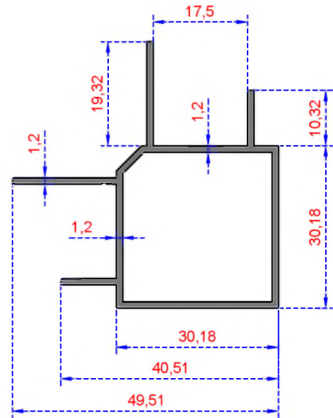
Sistem Kodu 2910 Ağırlık (kg/mt) 0,560
