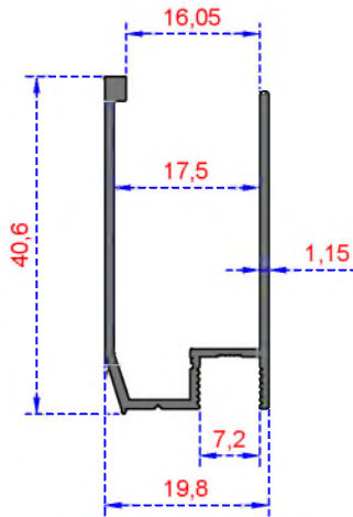
Sistem Kodu 2907 Ağırlık (kg/mt) 0,316
