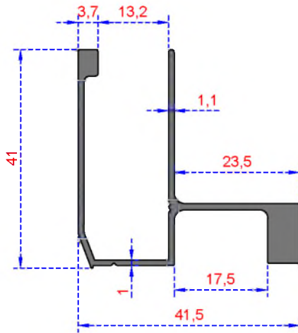
Sistem Kodu 2908 Ağırlık (kg/mt) 0,559
