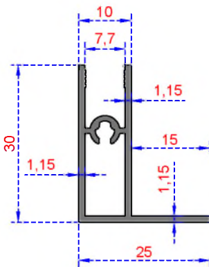
Sistem Kodu 2961 Ağırlık (kg/mt) 0,303
