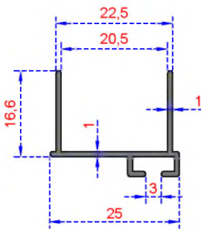
Sistem Kodu 1733 Ağırlık (kg/mt) 0,185
