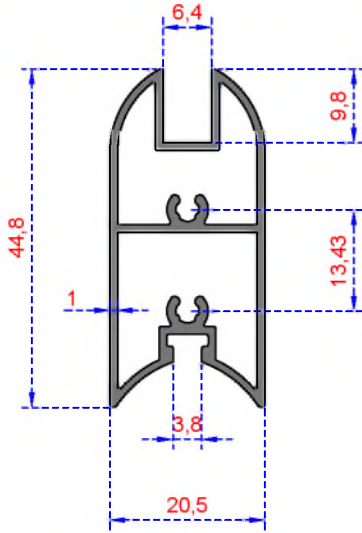
Sistem Kodu 2222 Ağırlık (kg/mt) 0,530
