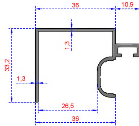
Sistem Kodu 2979 Ağırlık (kg/mt) 0,460
