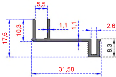
Sistem Kodu 2916 Ağırlık (kg/mt) 0,201
