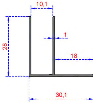
Sistem Kodu 2914 Ağırlık (kg/mt) 0,228
