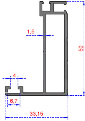
Sistem Kodu 505 Ağırlık (kg/mt) 0,631
