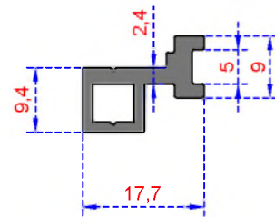
Sistem Kodu 507 Ağırlık (kg/mt) 0,256
