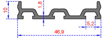
Sistem Kodu 510 Ağırlık (kg/mt) 0,395
