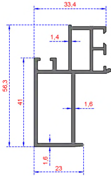
Sistem Kodu 504 Ağırlık (kg/mt) 0,835
