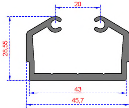
Sistem Kodu 513 Ağırlık (kg/mt) 0,865
