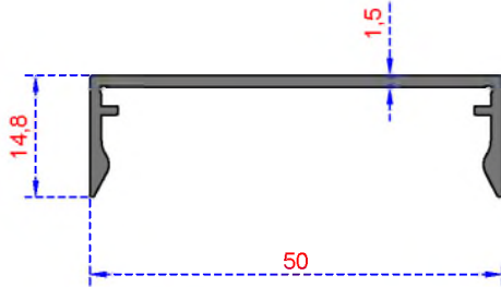
Sistem Kodu 509 Ağırlık (kg/mt) 0,325
