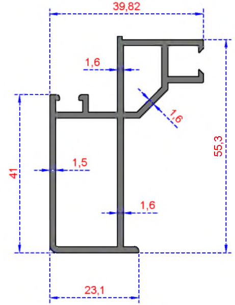
Sistem Kodu 506 Ağırlık (kg/mt) 0,835
