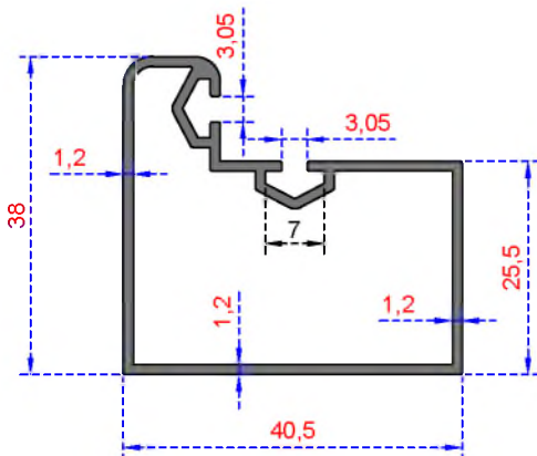
Sistem Kodu 219 Ağırlık (kg/mt) 0,552
