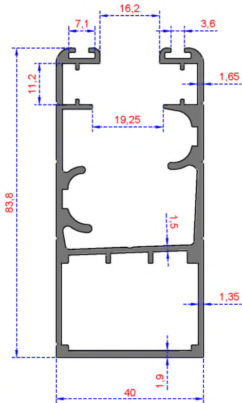
Sistem Kodu 228 Ağırlık (kg/mt) 1,556
