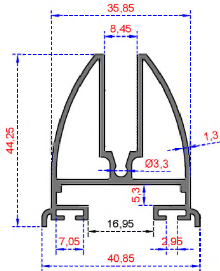
Sistem Kodu 221 Ağırlık (kg/mt) 0,820
