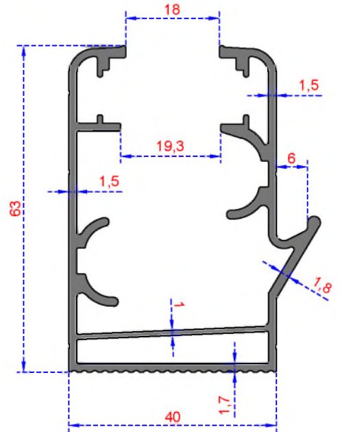
Sistem Kodu 238 Ağırlık (kg/mt) 1,199
