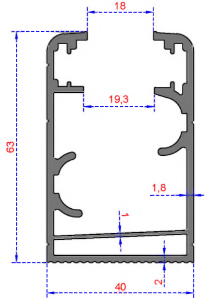
Sistem Kodu 199 Ağırlık (kg/mt) 1,325
