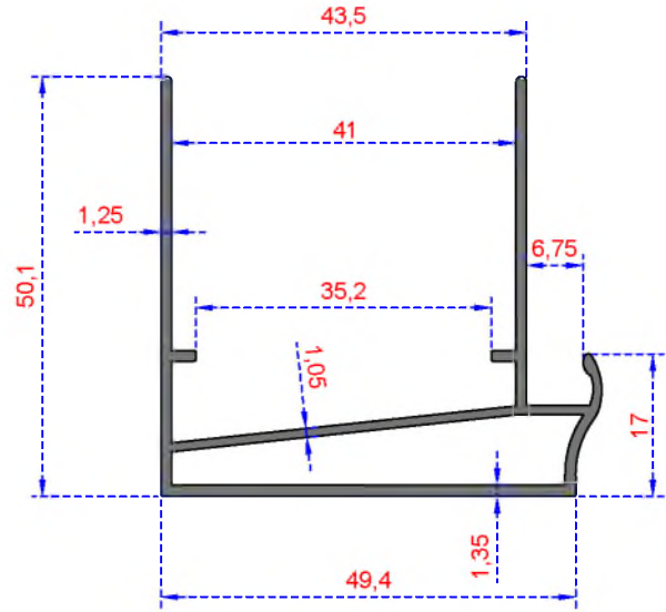
Sistem Kodu 257 Ağırlık (kg/mt) 0,700
