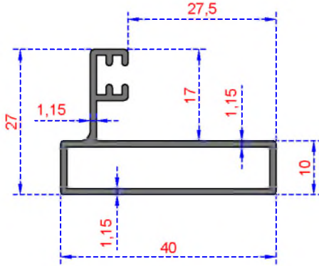
Sistem Kodu 204 Ağırlık (kg/mt) 0,410
