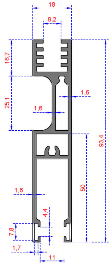
Sistem Kodu 211 Ağırlık (kg/mt) 1,245
