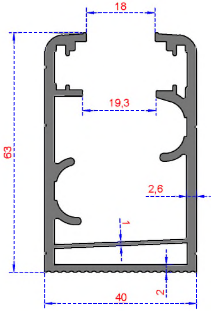
Sistem Kodu 200 Ağırlık (kg/mt) 1,495
