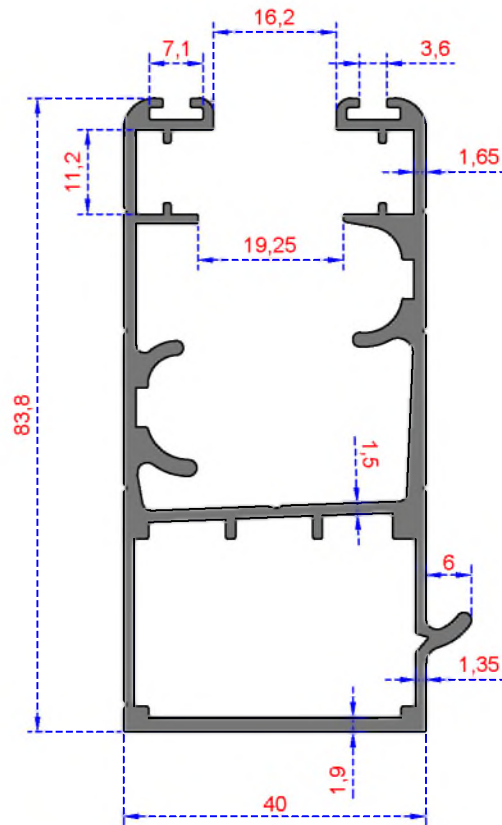
Sistem Kodu 229 Ağırlık (kg/mt) 1,592
