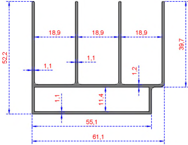
Sistem Kodu 254 Ağırlık (kg/mt) 0,900
