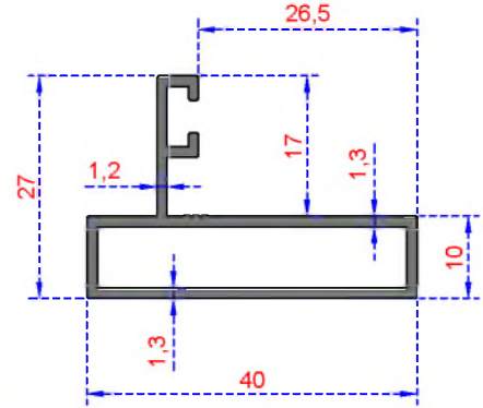
Sistem Kodu 225 Ağırlık (kg/mt) 0,430
