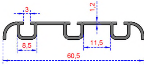
Sistem Kodu 256 Ağırlık (kg/mt) 0,365
