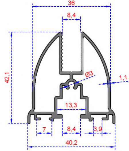
Sistem Kodu 240 Ağırlık (kg/mt) 0,702
