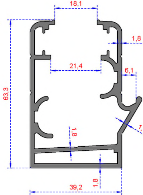
Sistem Kodu 216 Ağırlık (kg/mt) 1,372
