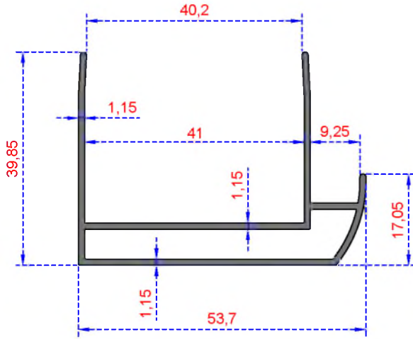
Sistem Kodu 214 Ağırlık (kg/mt) 0,583
