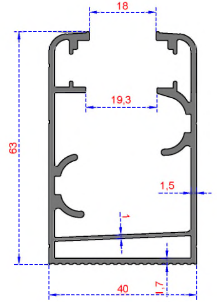
Sistem Kodu 239 Ağırlık (kg/mt) 1,128
