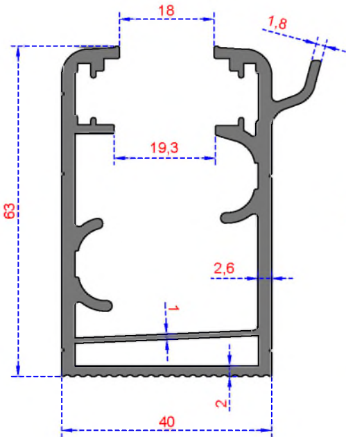
Sistem Kodu 201 Ağırlık (kg/mt) 1,565
