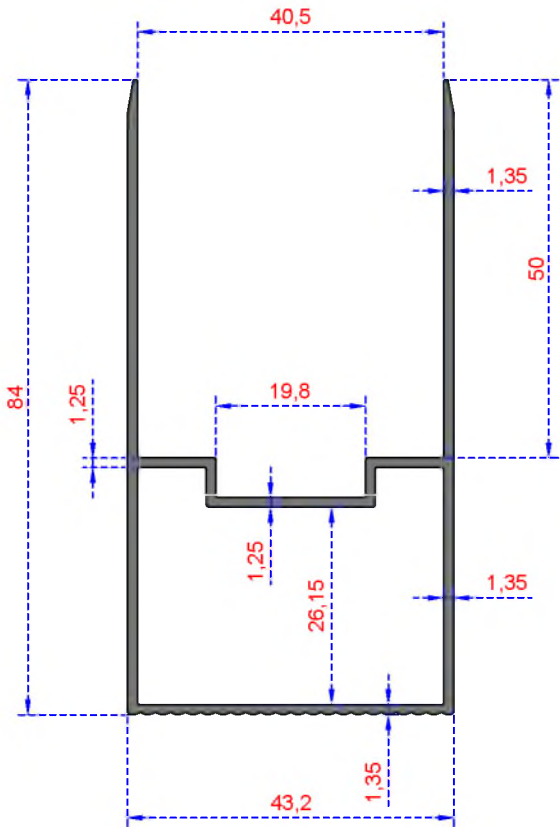
Sistem Kodu 215 Ağırlık (kg/mt) 0,910
