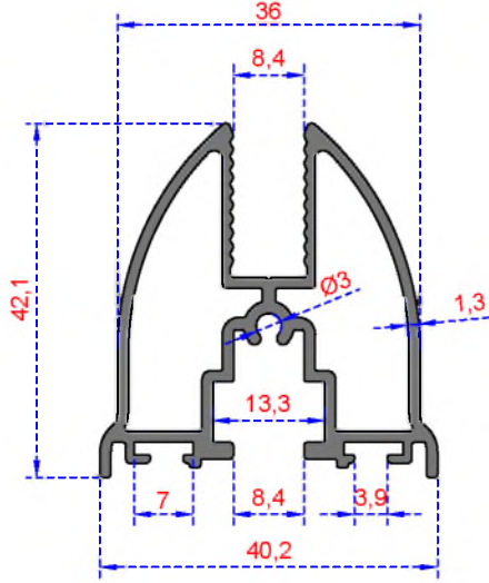
Sistem Kodu 202 Ağırlık (kg/mt) 0,812
