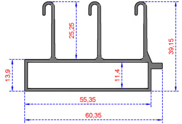
Sistem Kodu 255 Ağırlık (kg/mt) 0,845
