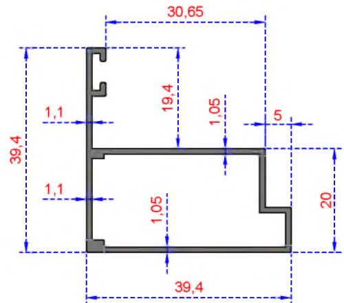
Sistem Kodu 227 Ağırlık (kg/mt) 0,430
