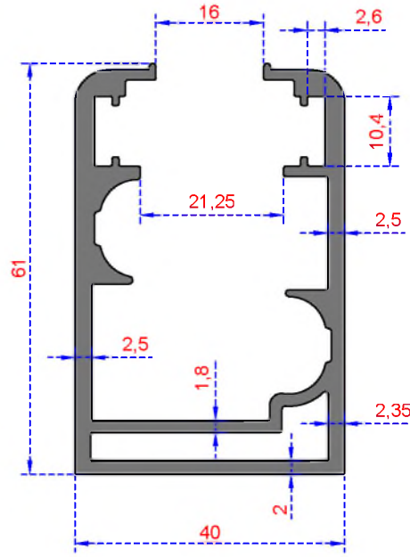
Sistem Kodu 7106 Ağırlık (kg/mt) 1,535
