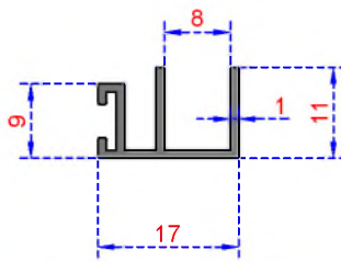
Sistem Kodu 206 Ağırlık (kg/mt) 0,136
