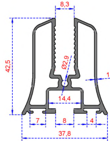
Sistem Kodu 245 Ağırlık (kg/mt) 0,745
