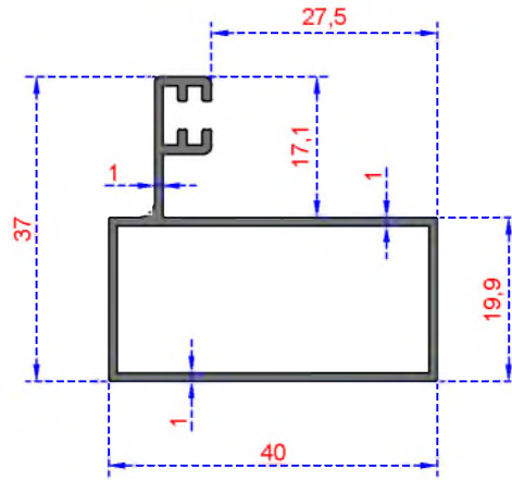
Sistem Kodu 233 Ağırlık (kg/mt) 0,420
