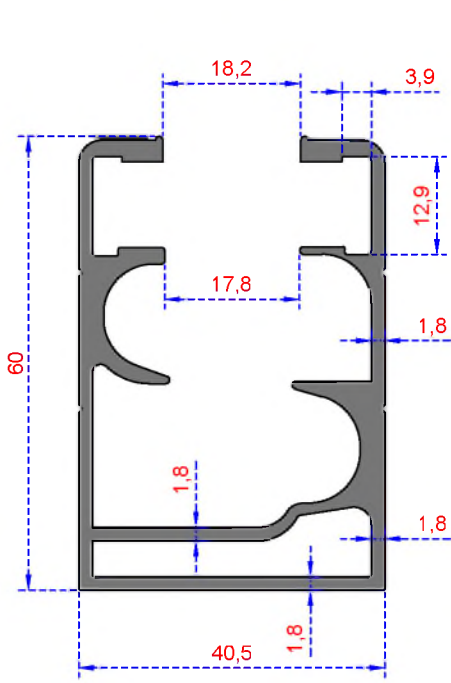
Sistem Kodu 220 Ağırlık (kg/mt) 1,425
