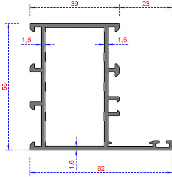
Sistem Kodu 8000 Ağırlık (kg/mt) 1,078
