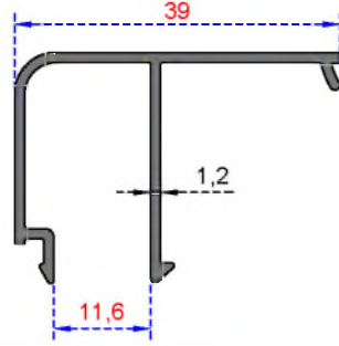
Sistem Kodu 4017 Ağırlık (kg/mt) 0,322
