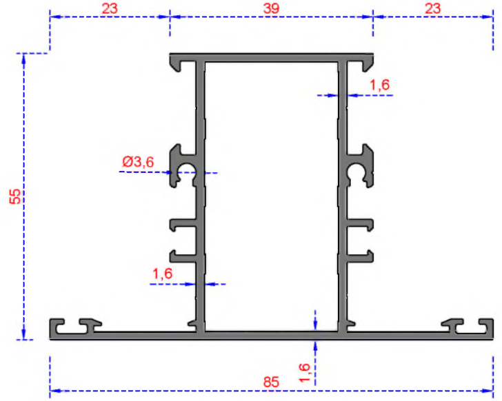
Sistem Kodu 8001 Ağırlık (kg/mt) 1,243
