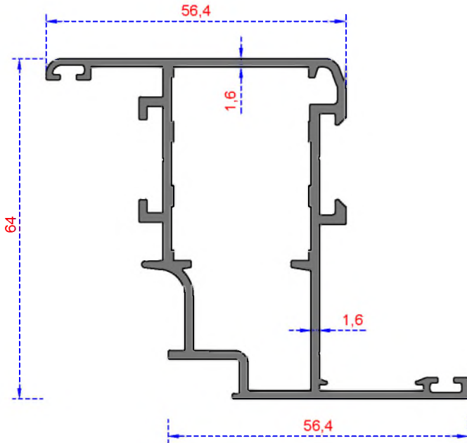
Sistem Kodu 8002 Ağırlık (kg/mt) 1,258
