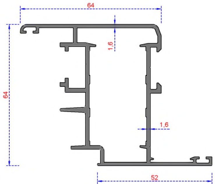
Sistem Kodu 8003 Ağırlık (kg/mt) 1,417
