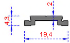
Sistem Kodu 614 Ağırlık (kg/mt) 0,130
