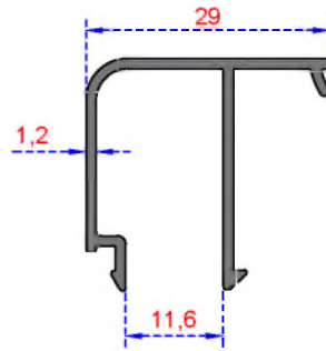
Sistem Kodu 4022 Ağırlık (kg/mt) 0,290
