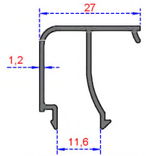
Sistem Kodu 4023 Ağırlık (kg/mt) 0,287
