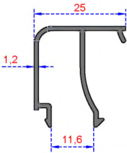
Sistem Kodu 4024 Ağırlık (kg/mt) 0,280
