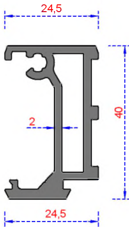
Sistem Kodu 4014 Ağırlık (kg/mt) 0,775
