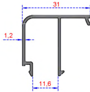
Sistem Kodu 4021 Ağırlık (kg/mt) 0,296
