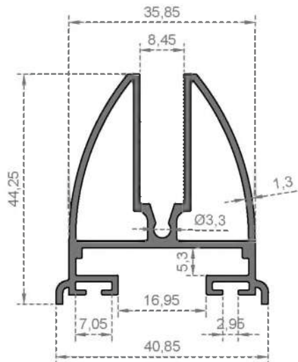
System Code 221 Weight (kg/mt) 0,820
