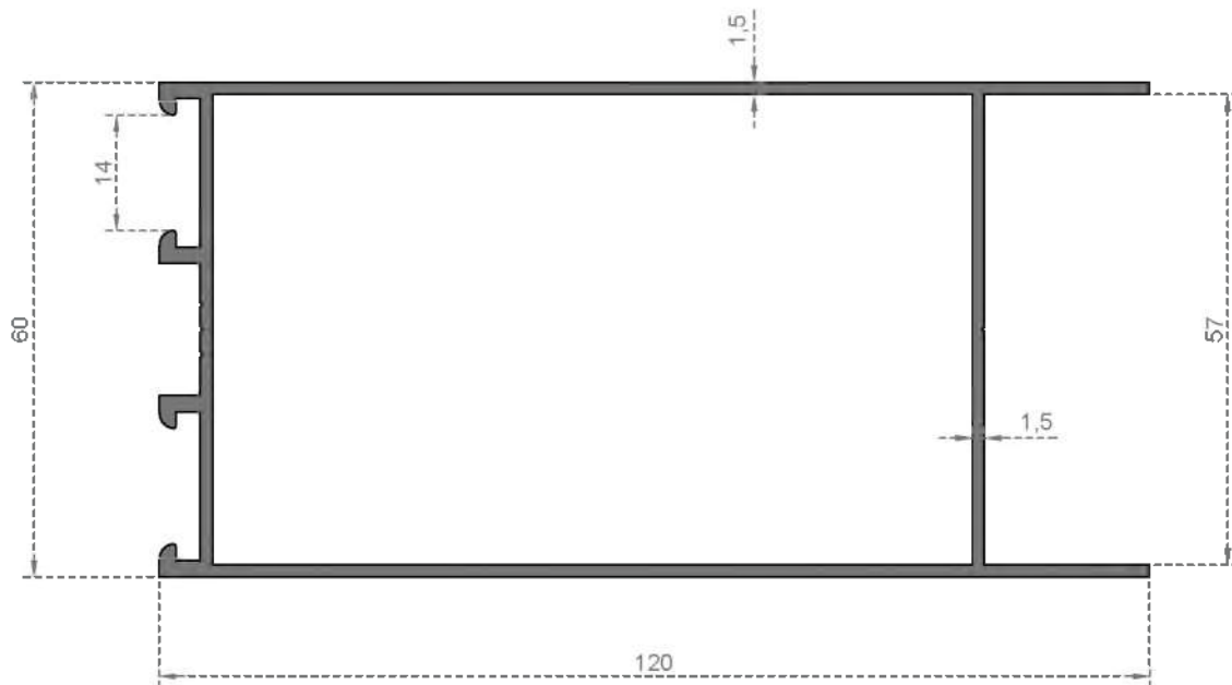
PLINTH
