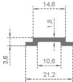
INNER ROD
