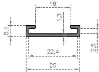
OUTER ROD
