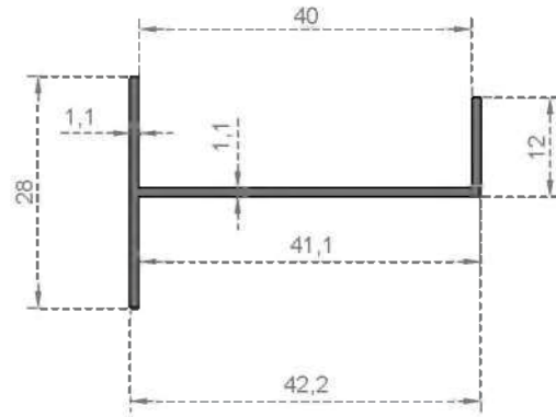
Sistem Kodu 7044 Ağırlık (kg/m) 0,240
