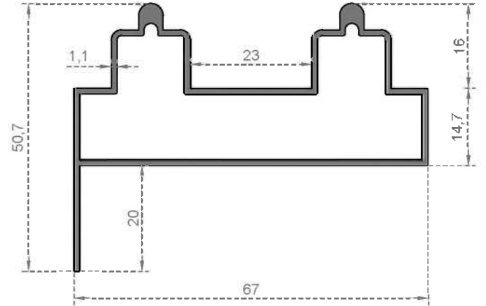
Sistem Kodu 401 Ağırlık (kg/mt) 0,741
