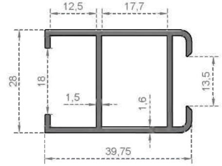
Sistem Kodu: 7506 Ağırlık (kg/mt): 0,605
