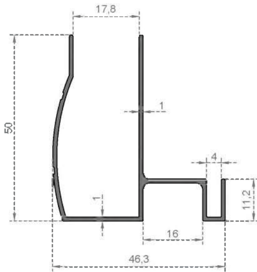
Sistem Kodu 2900 Ağırlık (kg/mt) 0,456
