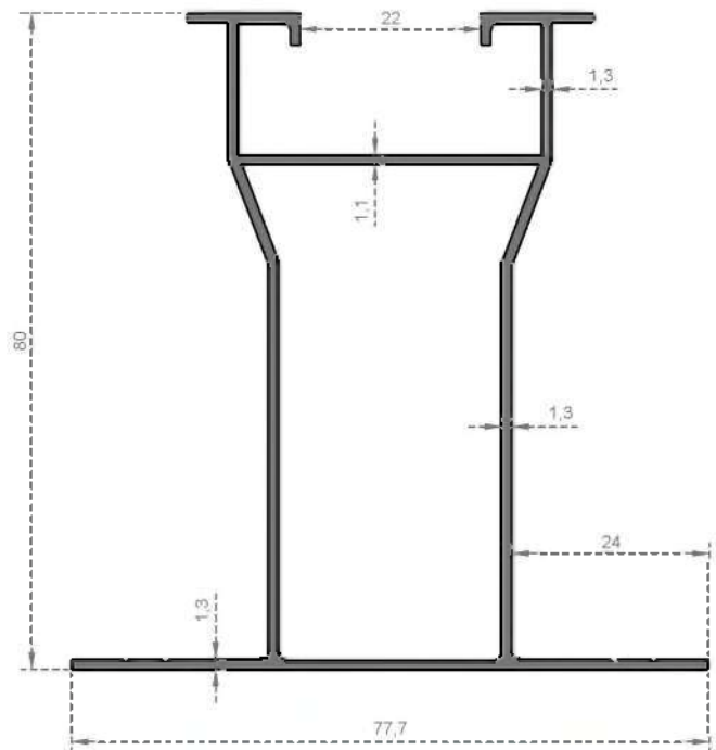
Sistem Kodu 49560 Ağırlık (kg/mt) 1,035
