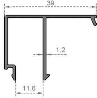
Sistem Kodu 4017 Ağırlık (kg/mt) 0,330
