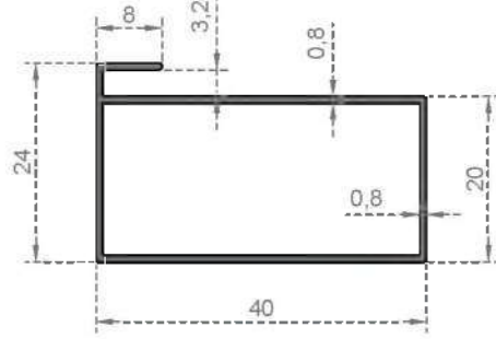
Sistem Kodu 803 Ağırlık (kg/mt) 0,278
