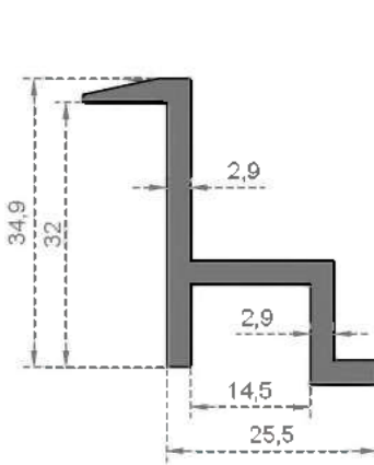
Sistem Kodu 6725 Ağırlık (kg/mt) 0,605
