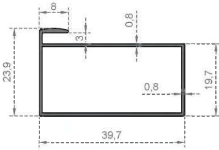
Sistem Kodu 802 Ağırlık (kg/mt) 0,280
