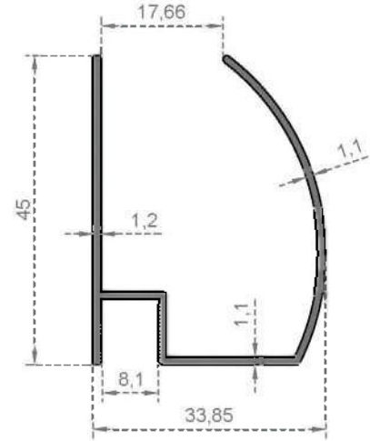
Sistem Kodu 2858 Ağırlık (kg/mt) 0,407
