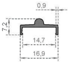
Sistem Kodu 5945 Ağırlık (kg/mt) 0,092
