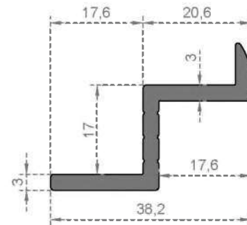
Sistem Kodu 6704 Ağırlık (kg/mt) 0,500
