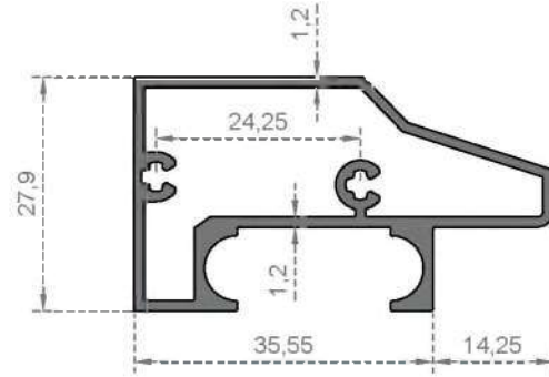
Sistem Kodu 2948 Ağırlık (kg/mt) 0,651
