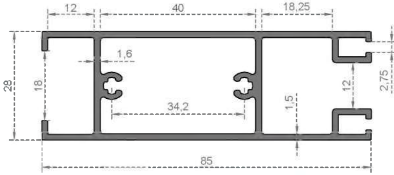
Sistem Kodu: 7505 Ağırlık (kg/mt): 1,215
