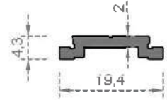
Sistem Kodu 614 Ağırlık (kg/m) 0,130
