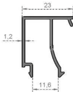
Sistem Kodu 4025 Ağırlık (kg/mt) 0,279
