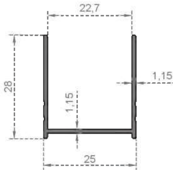
Sistem Kodu 1257 Ağırlık (kg/mt) 0,241
