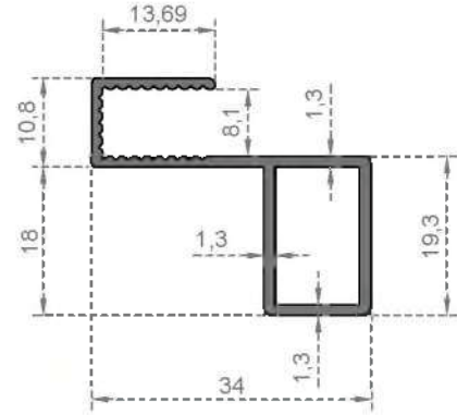
Sistem Kodu 235 Ağırlık (kg/mt) 0,360
