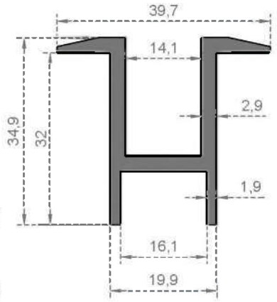
Sistem Kodu 6724 Ağırlık (kg/mt) 0,725
