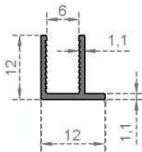
Sistem Kodu 2997 Ağırlık (kg/mt) 0,095
