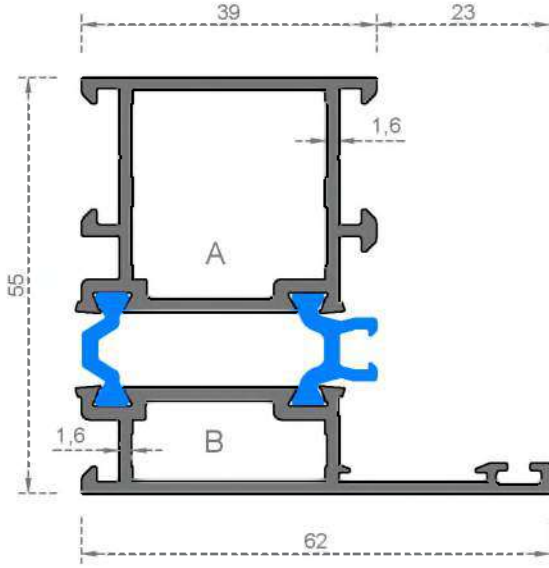
Sistem Kodu 4000 Ağırlık (kg/mt) 1,450
