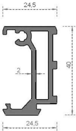
Sistem Kodu 4014 Ağırlık (kg/m) 0,775
