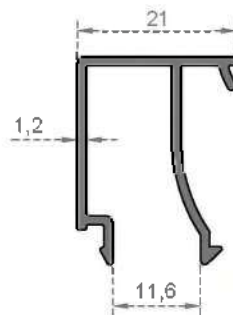
Sistem Kodu 4026 Ağırlık (kg/mt) 0,275
