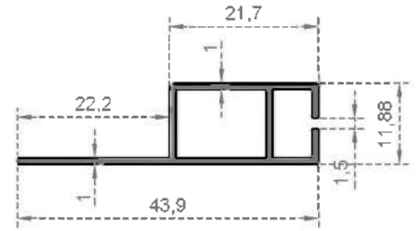
Sistem Kodu 2990 Ağırlık (kg/mt) 0,254
