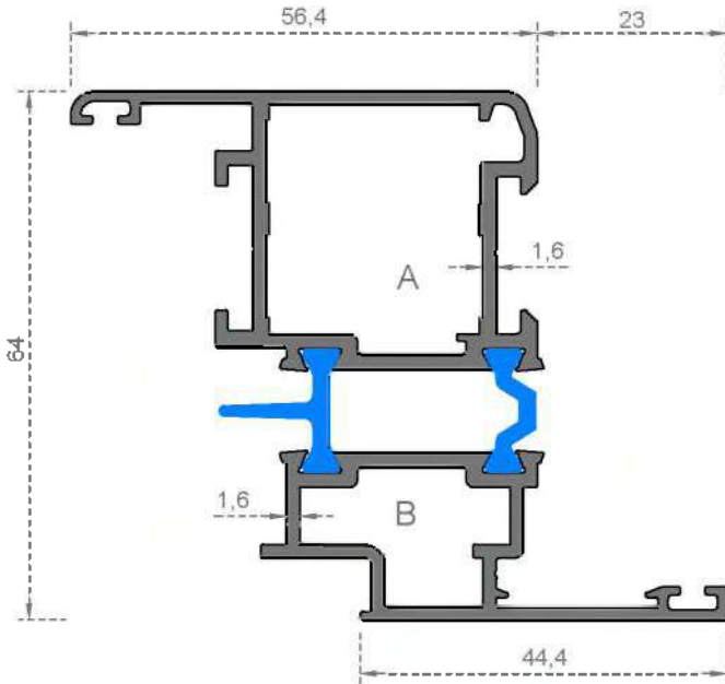
Sistem Kodu 4002 Ağırlık (kg/mt) 1,620
