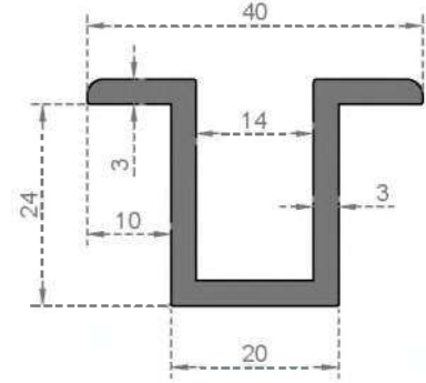
Sistem Kodu 6660 Ağırlık (kg/mt) 0,711
