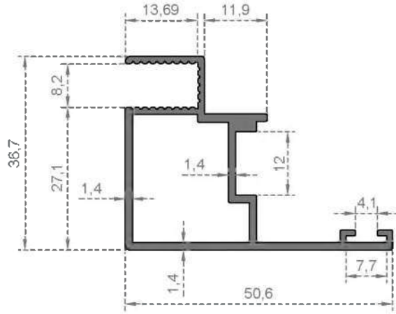
Sistem Kodu 234 Ağırlık (kg/mt) 0,615
