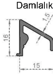
Sistem Kodu 8010 Ağırlık (kg/mt) 0,171
