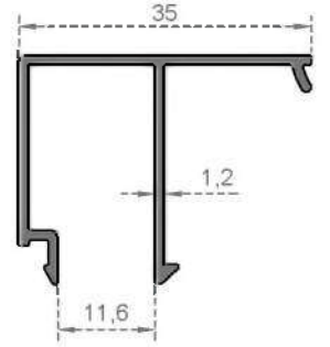
Sistem Kodu 4019 Ağırlık (kg/mt) 0,315
