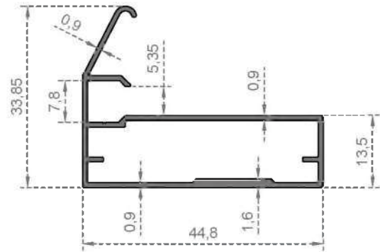
Sistem Kodu 832 Ağırlık (kg/mt) 0,401
