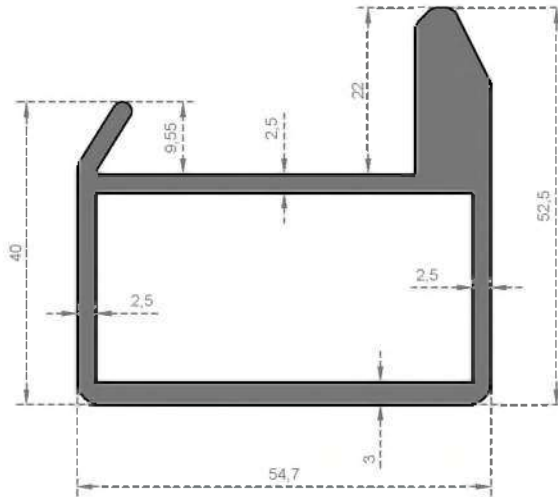
Sistem Kodu 6741 Ağırlık (kg/m 2 ) 1,740
