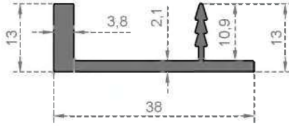
Sistem Kodu 808 Ağırlık (kg/mt) 0,372
