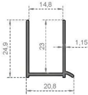
Sistem Kodu 2985 Ağırlık (kg/mt) 0,215
