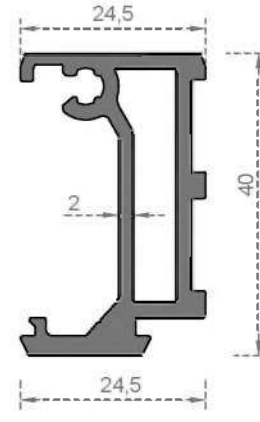
Sistem Kodu 4014 Ağırlık (kg/mt) 0,775
