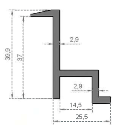
Sistem Kodu 6727 Ağırlık (kg/mt) 0,645
