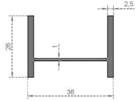
Sistem Kodu 6709 Ağırlık (kg/mt) 0,437
