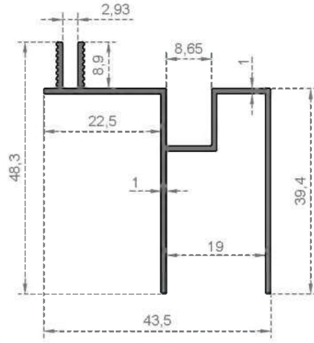
Sistem Kodu 2953 Ağırlık (kg/mt) 0,407
