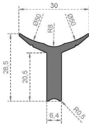
Sistem Kodu 7053 Ağırlık (kg/m) 0,545
