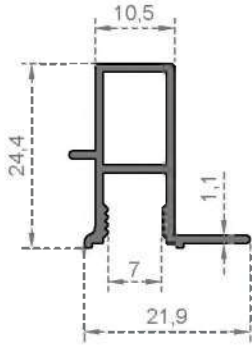
Sistem Kodu 1689 Ağırlık (kg/mt) 0,249
