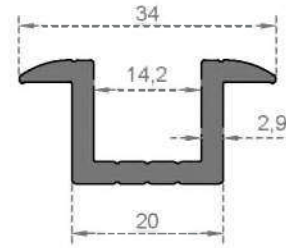
Sistem Kodu 6702 Ağırlık (kg/mt) 0,450
