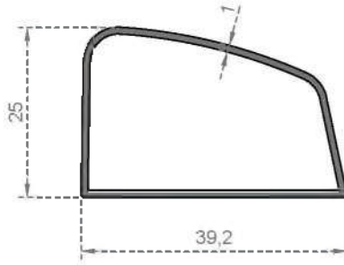
Sistem Kodu 2047 Ağırlık (kg/mt) 0,304
