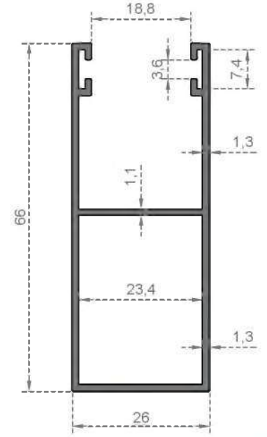
Sistem Kodu 5036 Ağırlık (kg/mt) 0,675
