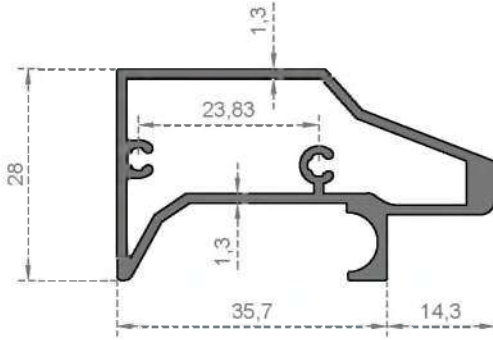
Sistem Kodu 2903 Ağırlık (kg/mt) 0,656
