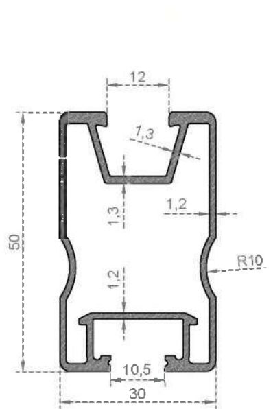
Sistem Kodu 6729 Ağırlık (kg/mt) 0,795
