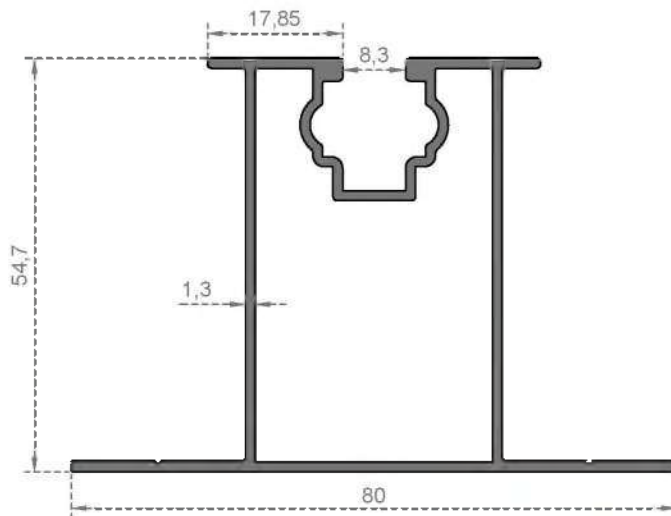
Sistem Kodu 6701 Ağırlık (kg/mt) 1,010
