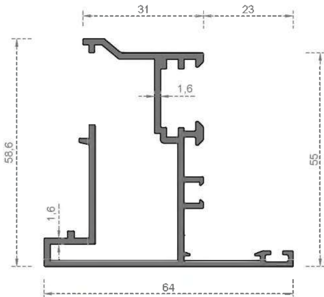
Sistem Kodu 8008 Ağırlık (kg/mt) 1,035
