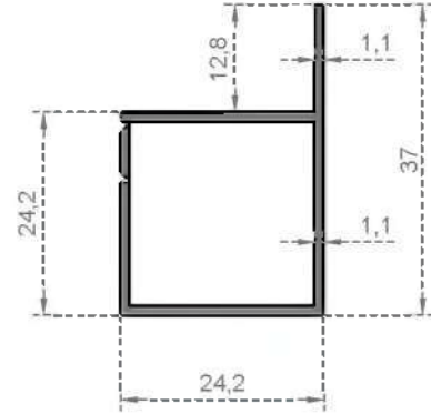
Sistem Kodu 2971 Ağırlık (kg/mt) 0,310
