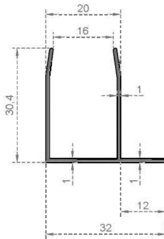
Sistem Kodu 2575 Ağırlık (kg/mt) 0,246
