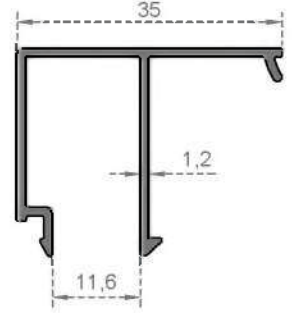
Sistem Kodu 4019 Ağırlık (kg/mt) 0,315
