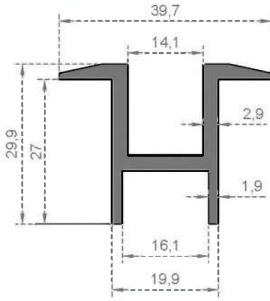
Sistem Kodu 6722 Ağırlık (kg/mt) 0,645
