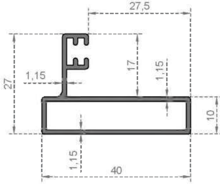
Sistem Kodu 204 Ağırlık (kg/mt) 0,410
