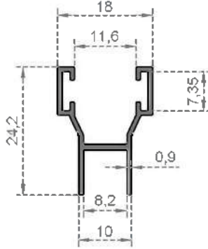
Sistem Kodu 205 Ağırlık (kg/mt) 0,185
