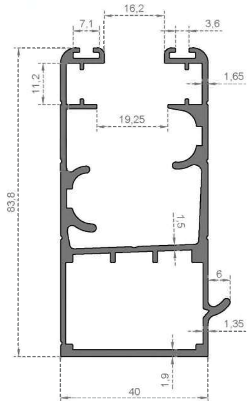
Sistem Kodu 229 Ağırlık (kg/mt) 1.597
