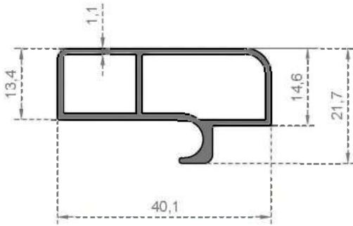
Sistem Kodu 2970 Ağırlık (kg/mt) 0,390
