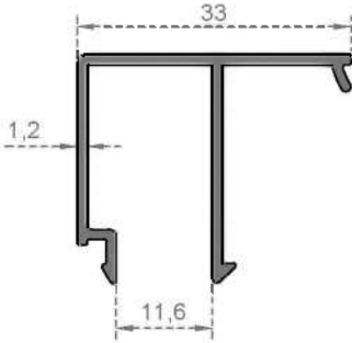
Sistem Kodu 4020 Ağırlık (kg/mt) 0,308
