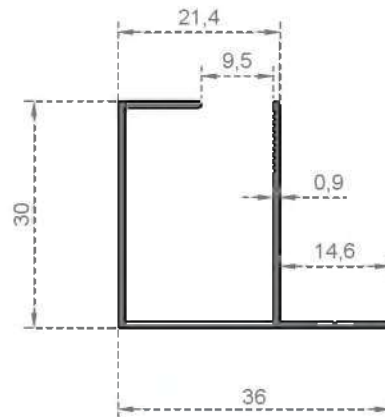
Sistem Kodu 2938 Ağırlık (kg/mt) 0,252
