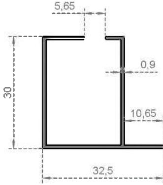
Sistem Kodu 2989 Ağırlık (kg/mt) 0,256
