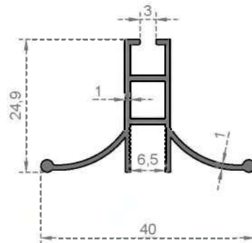
Sistem Kodu 2973 Ağırlık (kg/mt) 0,285
