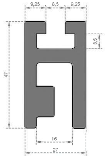
Sistem Kodu 6742 Ağırlık (kg/mt) 2,050
