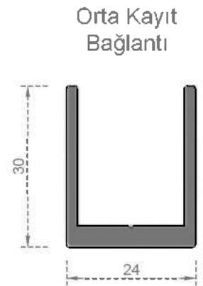
Sistem Kodu 8011 Ağırlık (kg/m) 0,545
