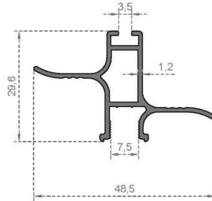
Sistem Kodu 1508 Ağırlık (kg/mt) 0,386
