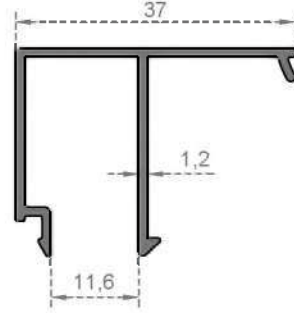
Sistem Kodu 4018 Ağırlık (kg/mt) 0,321
