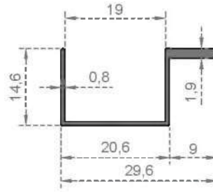
Sistem Kodu 829 Ağırlık (kg/mt) 0,151
