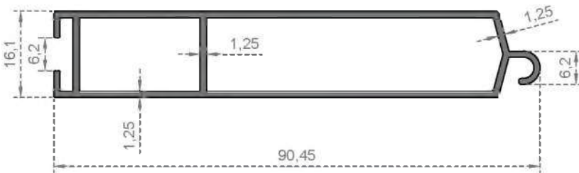
Sistem Kodu 5024 Ağırlık (kg/mt) 0,760
