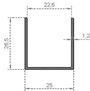
Sistem Kodu 2988 Ağırlık (kg/mt) 0,245
