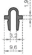
Sistem Kodu 5699 Ağırlık (kg/mt) 0,100
