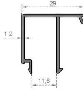
Sistem Kodu 4022 Ağırlık (kg/mt) 0,295
