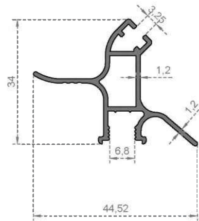
Sistem Kodu 1945 Ağırlık (kg/mt) 0,419
