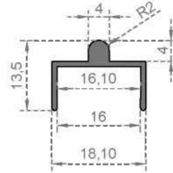
Sistem Kodu 6944 Ağırlık (kg/mt) 0,135
