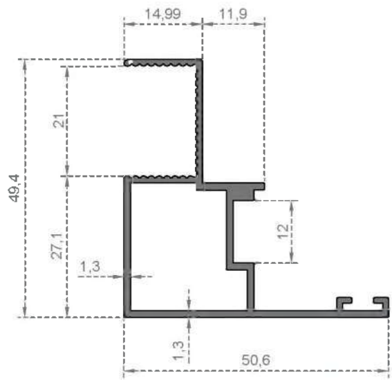
Sistem Kodu 242 Ağırlık (kg/mt) 0,618
