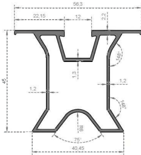
Sistem Kodu 6740 Ağırlık (kg/mt) 0,805
