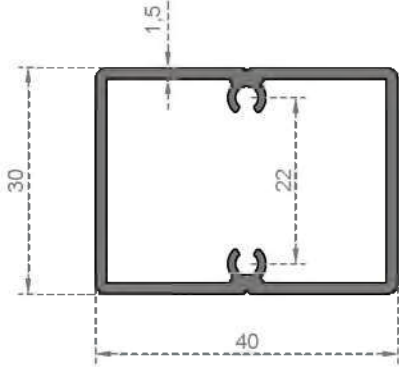
Sistem Kodu 6708 Ağırlık (kg/mt) 0,600
