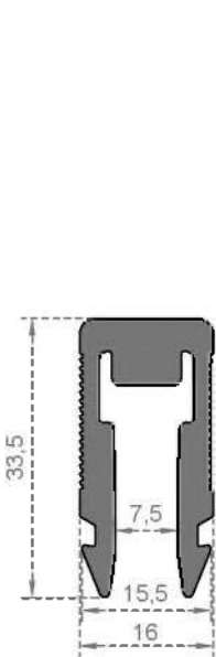
Sistem Kodu 6733 Ağırlık (kg/mt) 0,742
