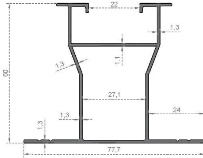
Sistem Kodu 6700 Ağırlık (kg/mt) 0,895
