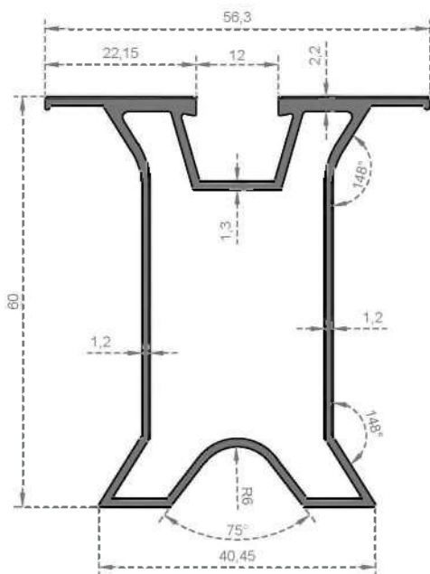
Sistem Kodu 6743 Ağırlık (kg/mt) 0,900
