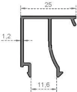
Sistem Kodu 4024 Ağırlık (kg/mt) 0,286
