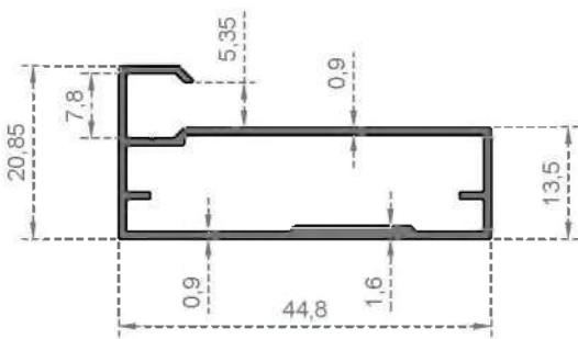
Sistem Kodu 831 Ağırlık (kg/mt) 0,358
